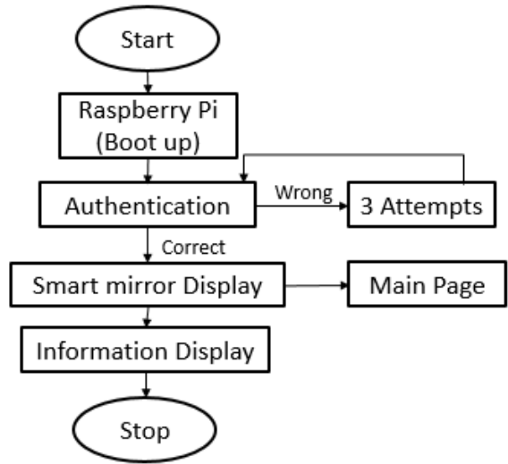
Fig 3. Login module
